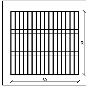
5 Detalhe Boca de Lobo - Grelha Sem Escala
