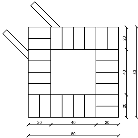
4 Detalhe Boca de Lobo - Dimenssões Sem Escala
