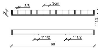
6 Detalhe Boca de Lobo - Dimenssões Grelha Sem Escala
